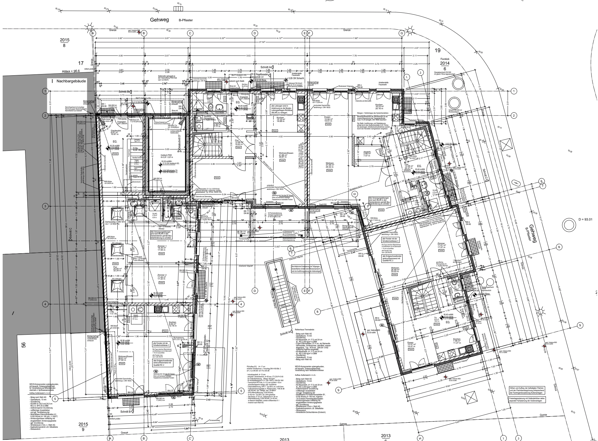
Erdgeschoss M 1 : 50
